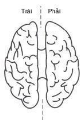
Bán cầu não trái và phải được liên kết bởi thể chai
