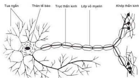
Sơ đồ đơn giản hóa một tế bào neuron thần kinh điển hình. Tín hiệu điện nhận được từ các tế bào khác qua các tua ngán
